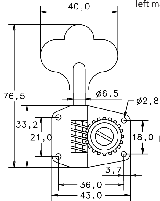
Vorderansicht front view
