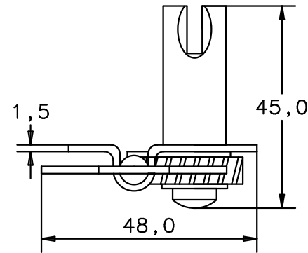
Draufsicht top view
