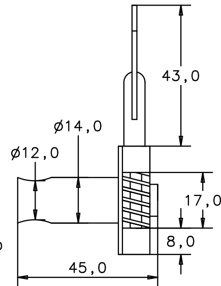
Seitenansicht von links side view left
