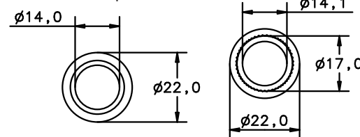
Draufsicht / Untersicht top view / bottom view
