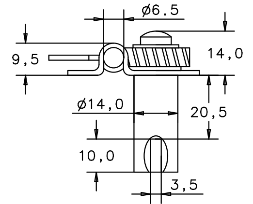
Untersicht bottom view
